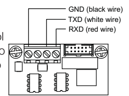
SA-232 wiring
