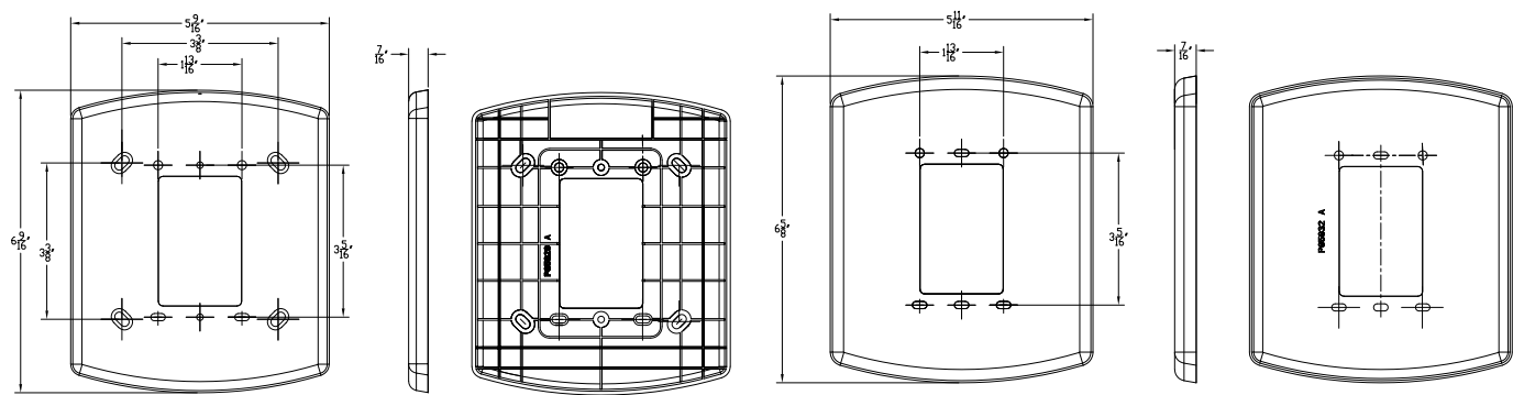
Figure 1. ELTP-SG
