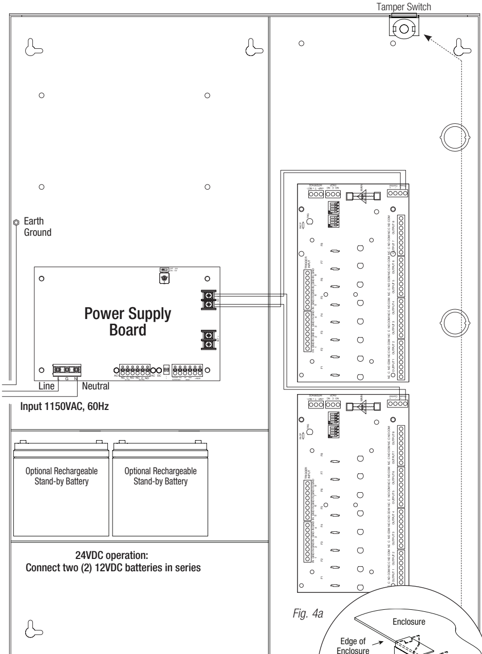
Fig. 4 - Maximal7D
