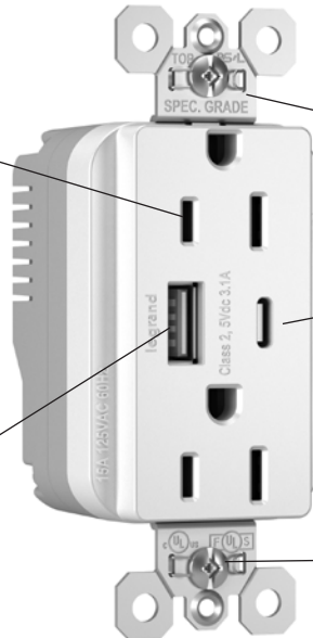
PTTR15ACUSBW
