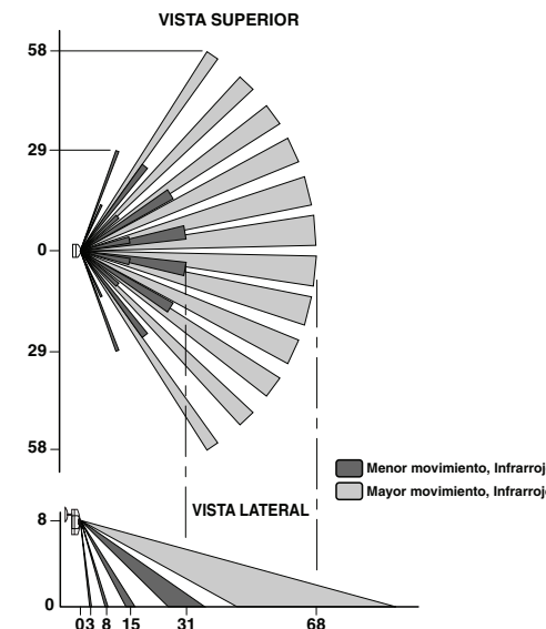
Figura 4 (No. de Cat. OSWVV) Rangos del Campo de Visión
