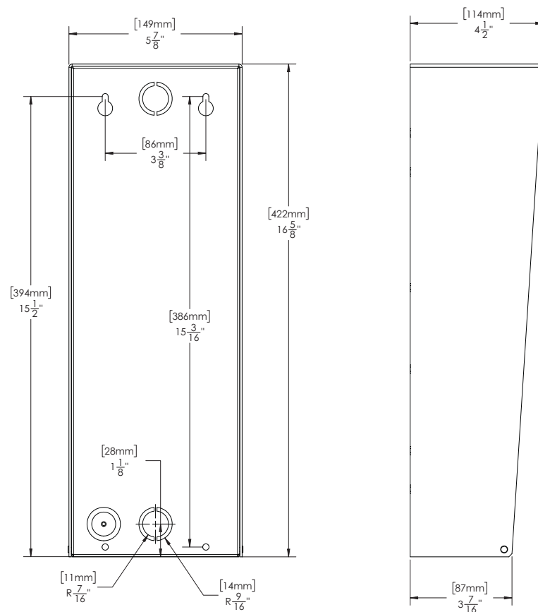
Figure 7 TX3-200-4U-C, TX3-1000-4U-C, TX3-2000-4U-C Dimensions
