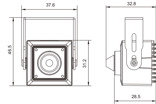
Figure 2-3 Dimensions (Pinhole lens)
