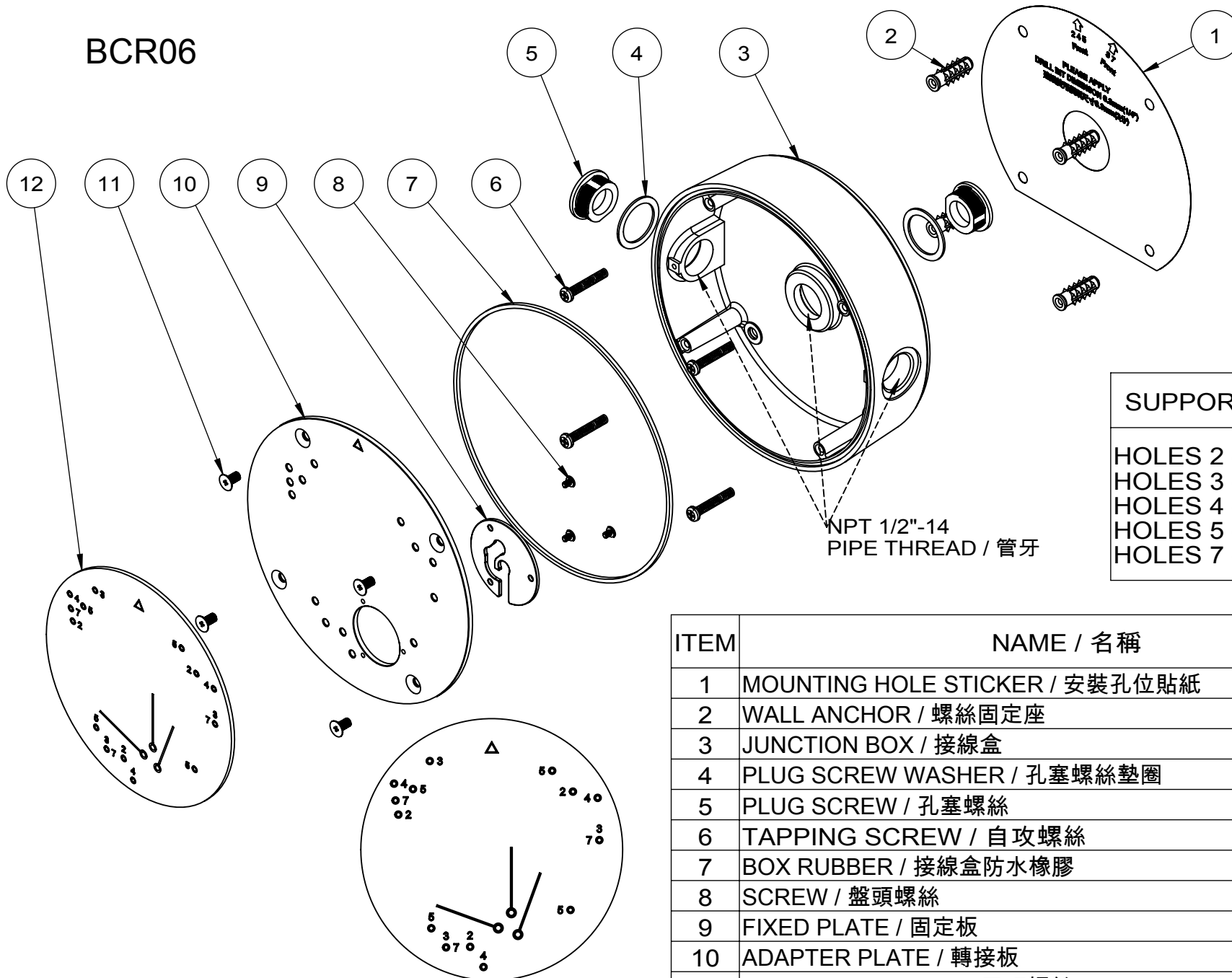
HOLE POSITION DIAGRAM 孔位圖
