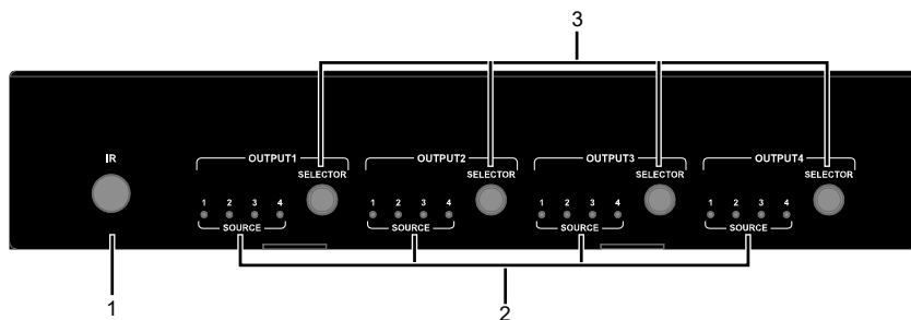
Panneau avant
