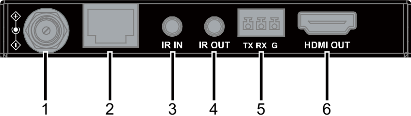
Panneau arrière
