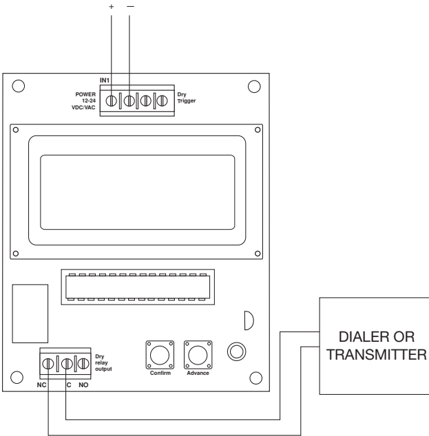
Fig. 8 - Test Timer:
