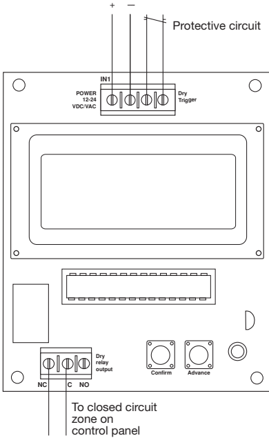
Fig. 4 - Delay Timer:
