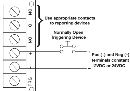
Fig. 4 - Delay Timer:
