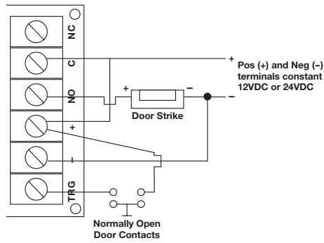
Fig. 5 - Timed Door Strike:
