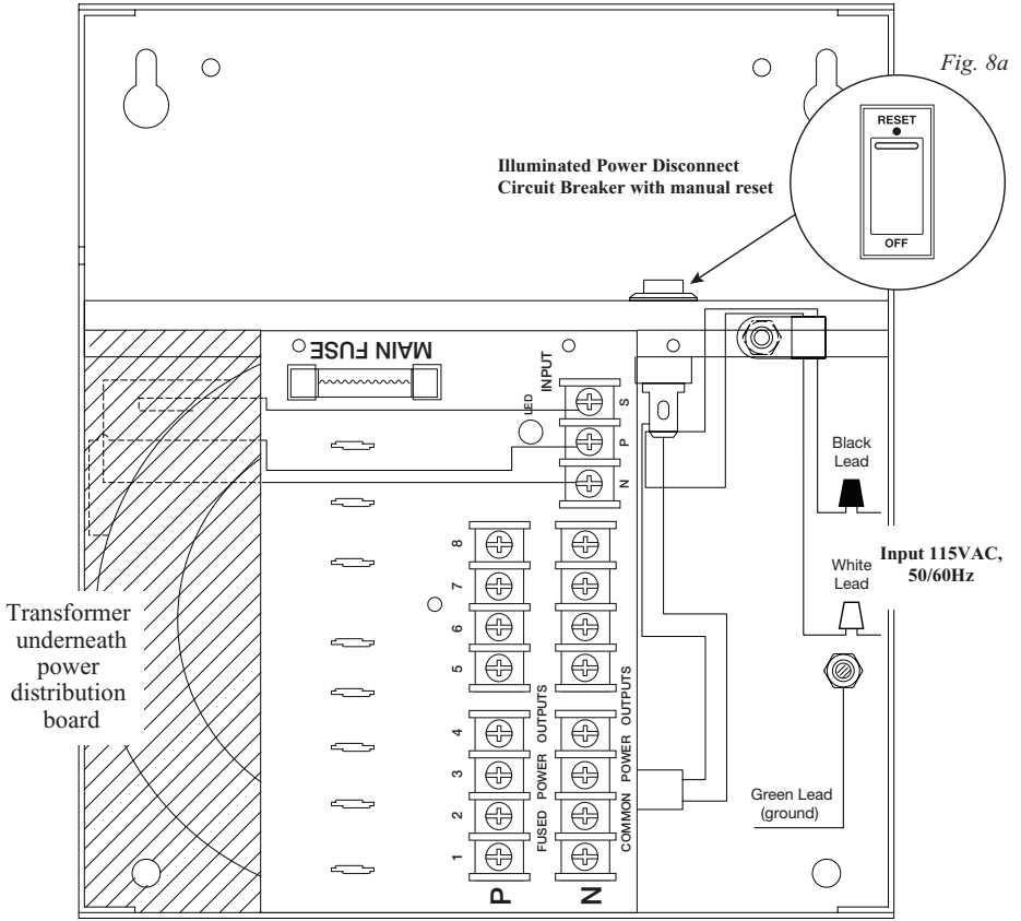
Fig. 8 - ALTV248300ULCBM
