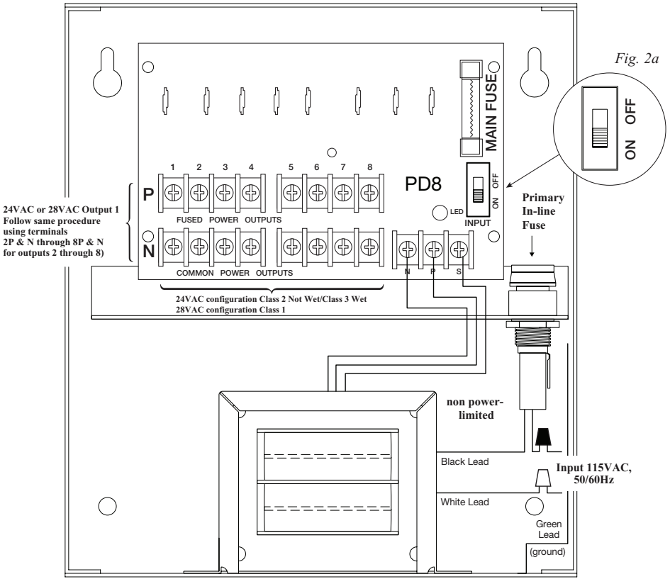
Fig. 2 - ALTV248ULCB
