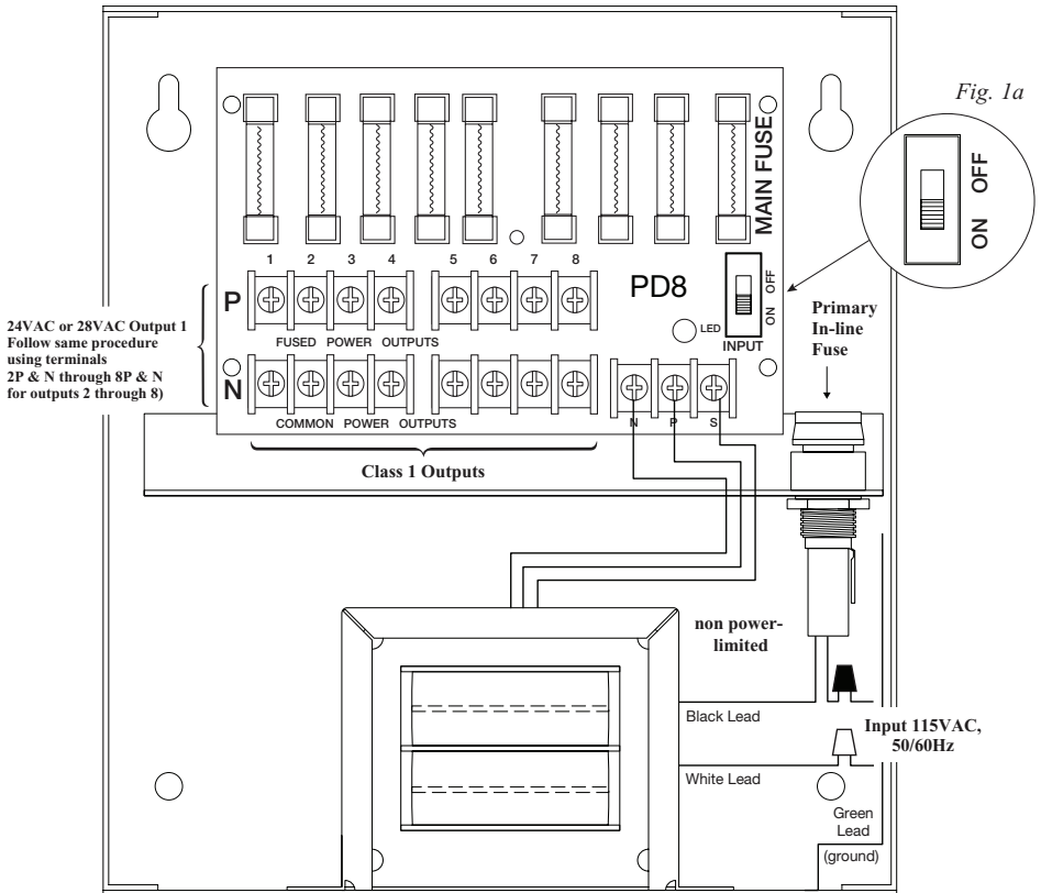
Fig. 1 - ALTV248UL
