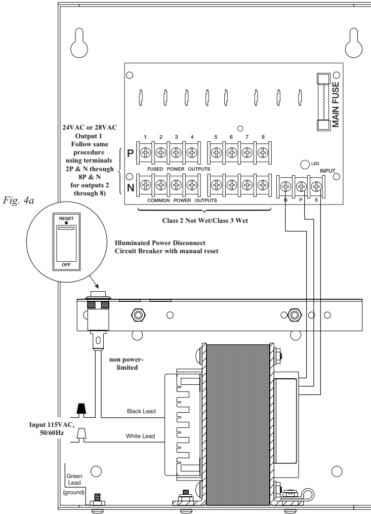
Fig. 4 - ALTV248175ULCB
