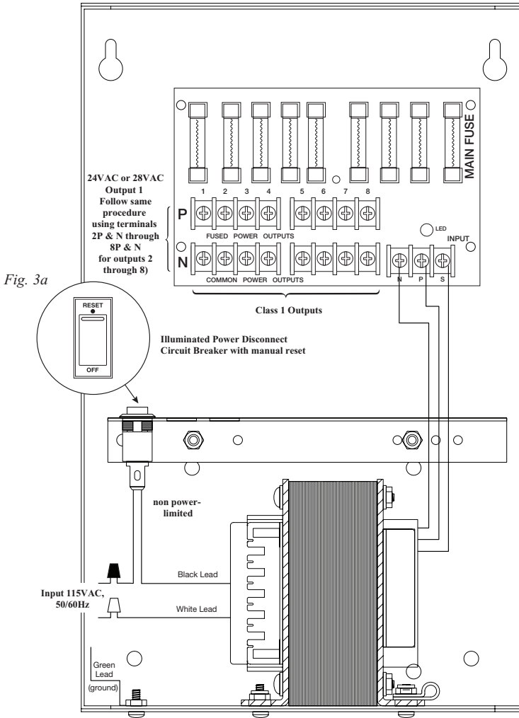
Fig. 3 - ALTV248175UL
