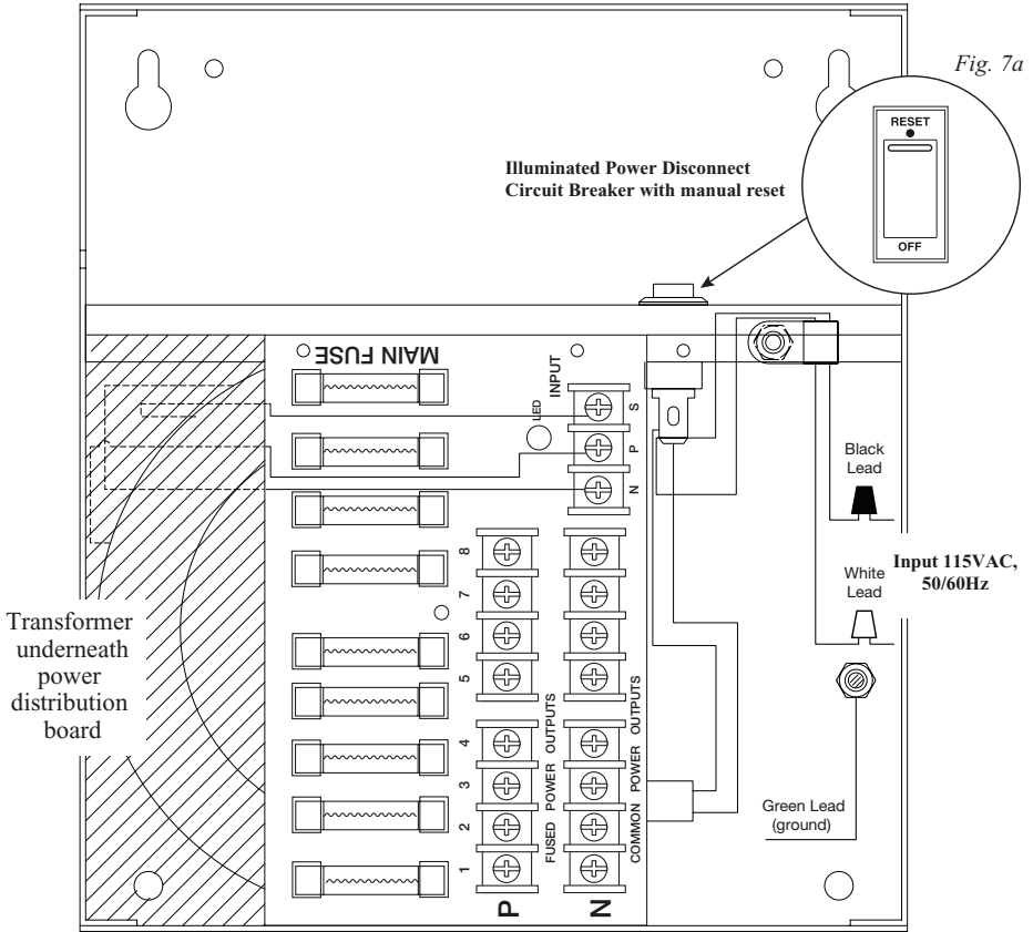
Fig. 7 - ALTV248300ULM
