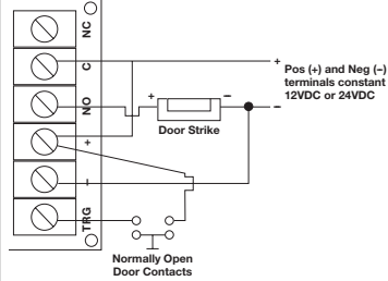
Fig. 5 - Timed Door Strike:
