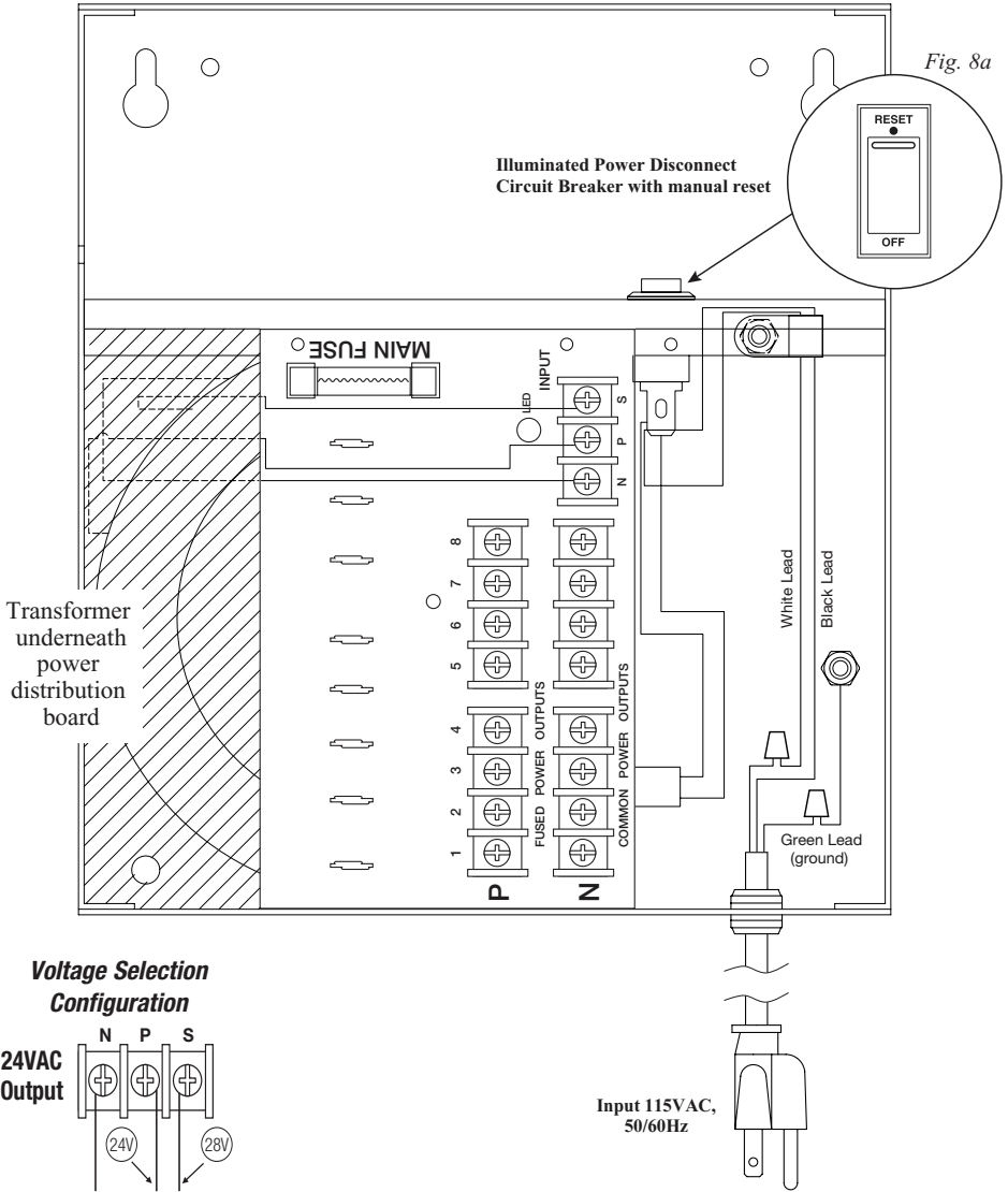
Fig. 8 - ALTV248300ULCBM3
