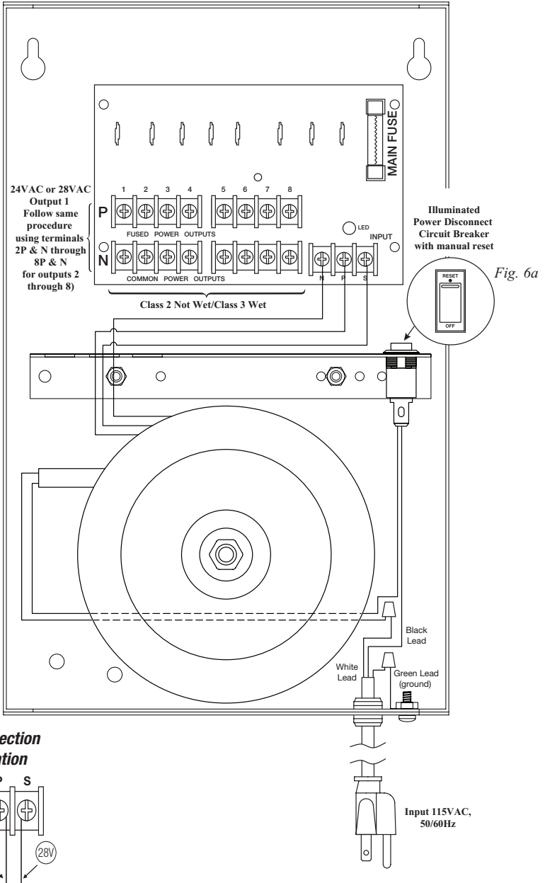
Fig. 6 - ALTV248300ULCB3
