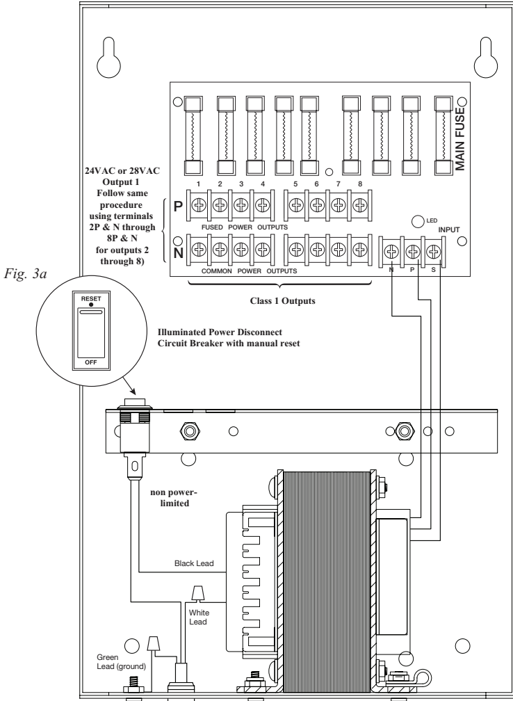
Fig. 3 - ALTV248175UL3
