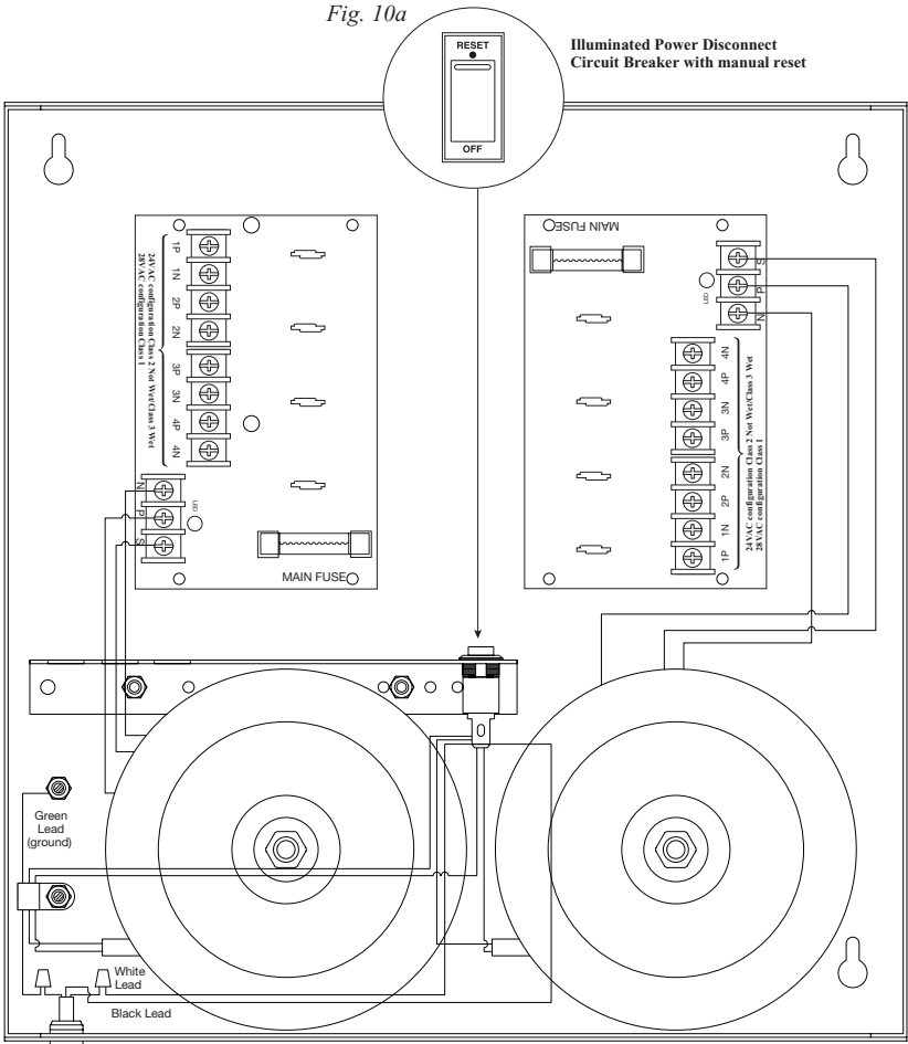
Fig. 10 - ALTV248600ULCB3
