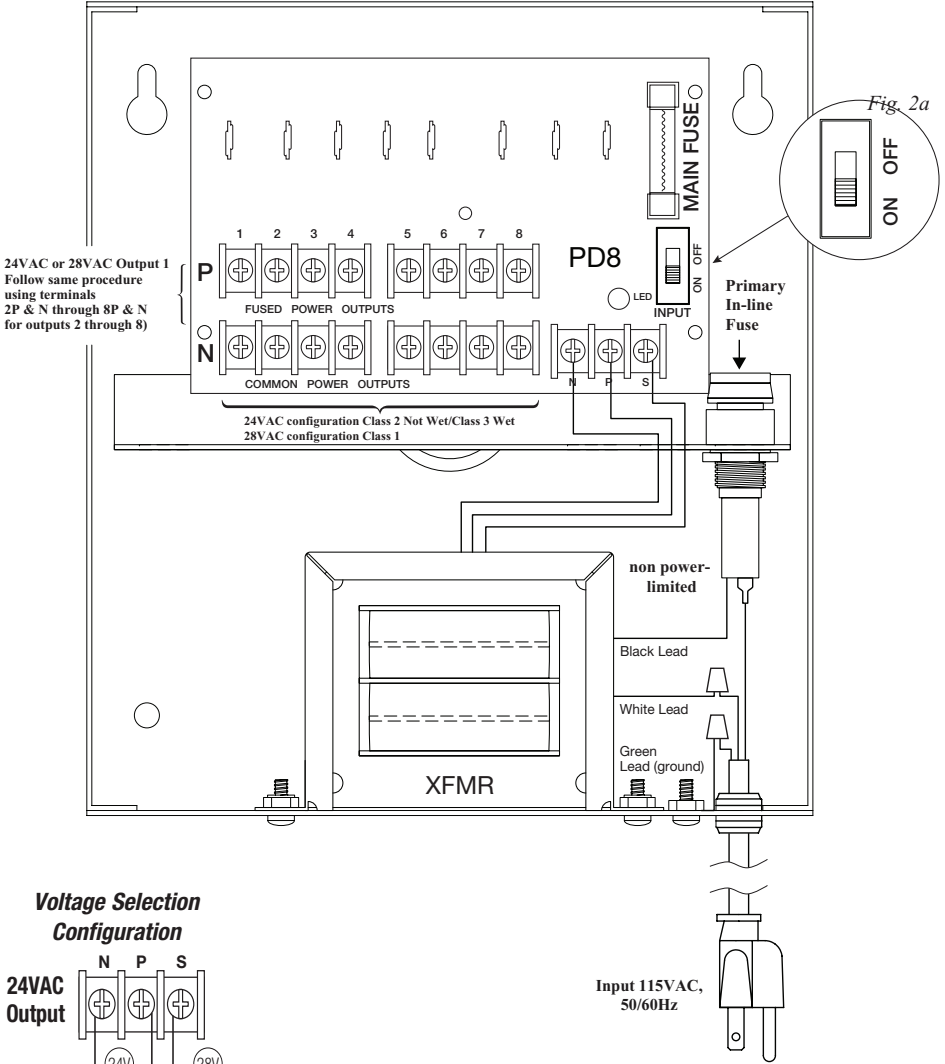
Fig. 2 - ALTV248ULCB3
