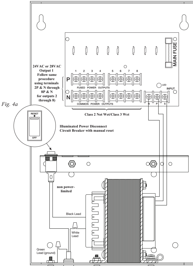
Fig. 4 - ALTV248175ULCB3
