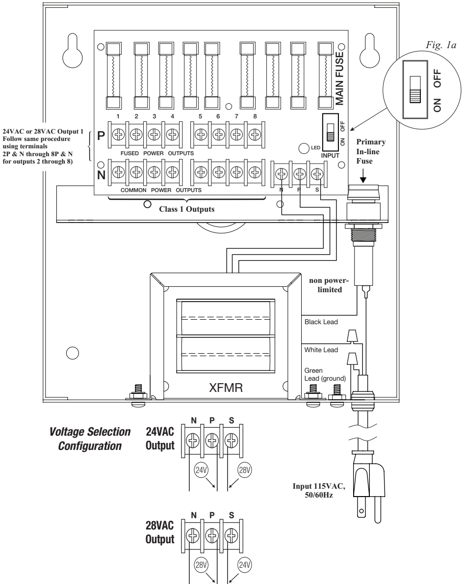
Fig. 1 - ALTV248UL3
