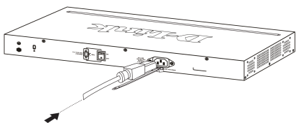
Insira o cabo de energia no switch
