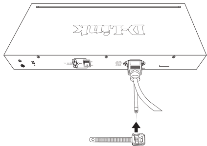
Conecte el retenedor a la abrazadera
