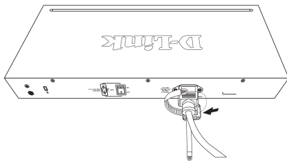
Enrole o suporte em volta do cabo de energia
