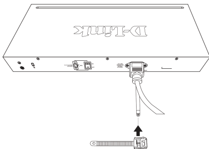
Conecte o suporte na braçadeira
