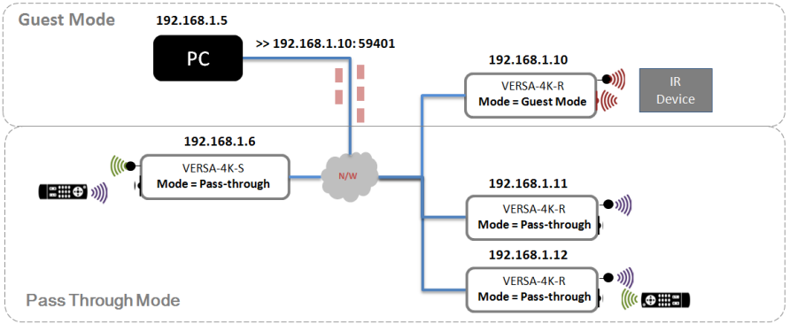
Fig 16. IR Over IP
