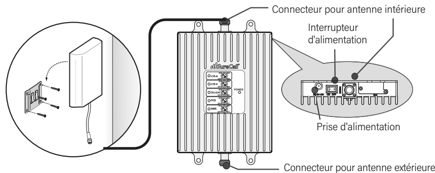
Diagramme de composants de l'amplificateur
