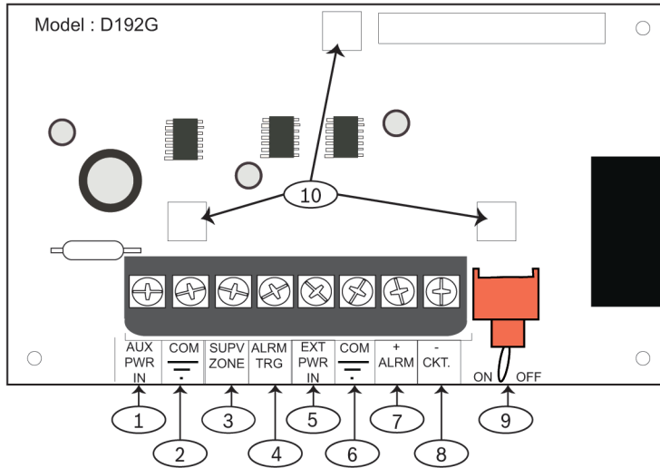
Figure 2.1: D192G_NAC_Module
