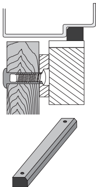
CX-AL004/CX-AL014 Spacer Bar
