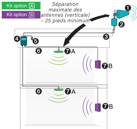
Aperçu de l'Installation
