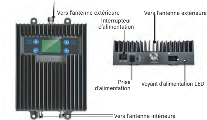
Diagramme de l'Unité Hôte
