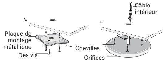
Installation de l'antenne UltraThin, option de montage 2x
