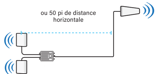
Maximiser la séparation entre les antennes
