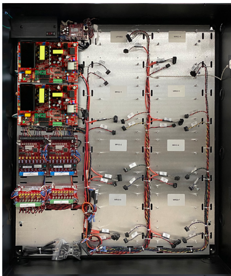
E8M2 Tie wrap
